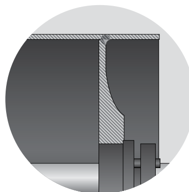
Preparación para soldadura del disco lateral biselado y soldado con arco sumergido para asegurar la máxima penetración de la soldadura
