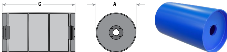
Poleas de Tambor de Servicio Minero - Sin Recubrimiento
