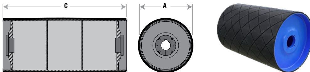
Poleas Profiled End Disc – Recubrimiento Diamantado
