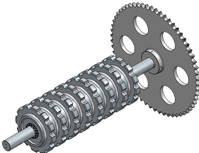
Sprockets Roller con Sprocket Motriz
